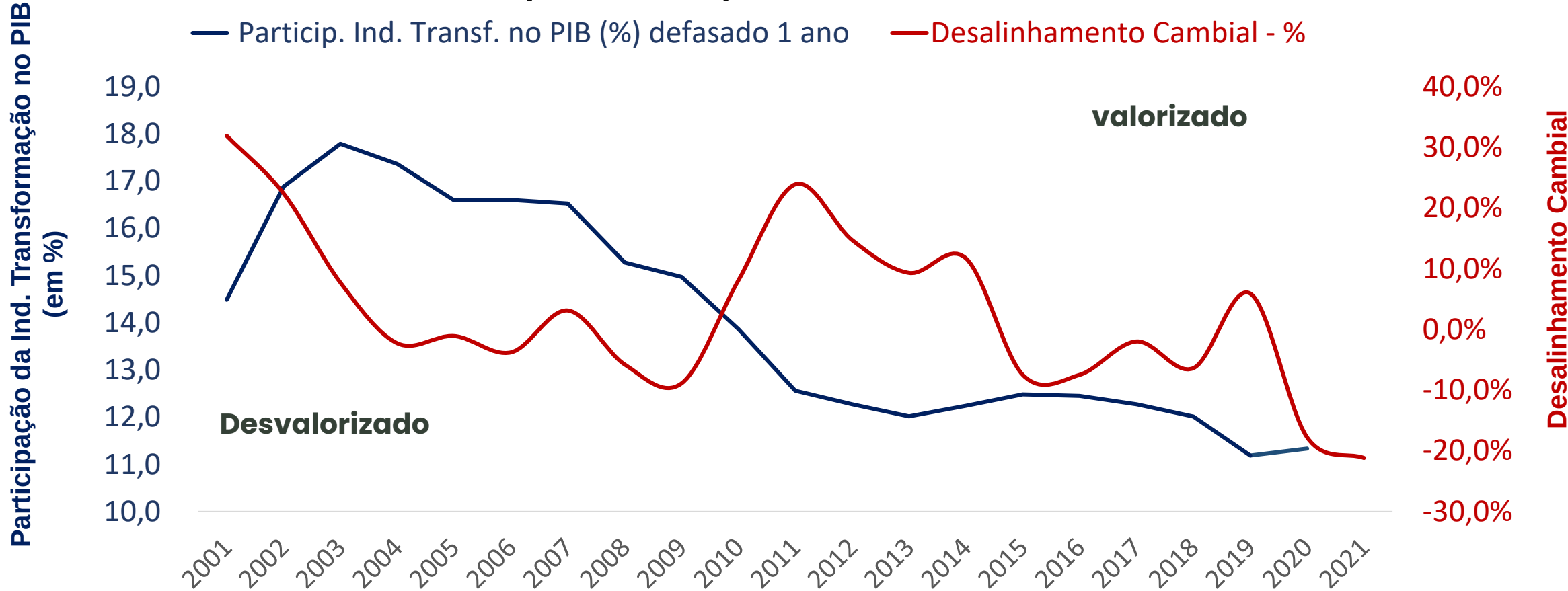
Desalinhamento Cambial 1 e Participação da Ind. Transformação no PIB (2001 – 2021) defasado em 1 ano
